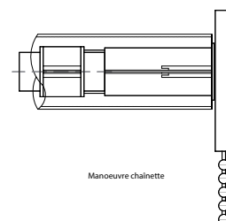
MANŒUVRE CHÂINETTE POUR LES COFFRES 70 ET 90 UNIQUEMENT (STORE INTÉRIEUR)
