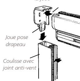
Clipage du coffre sur la joue
