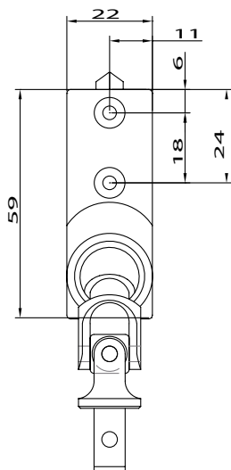
Renvoi à 45°
