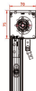
Coffre 70 manœuvre manuelle sortie verticale
