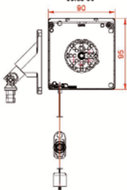
Coffre 90 manœuvre manuelle sortie 90°
