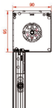
Coffre 90 manœuvre électrique
